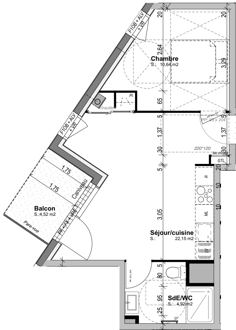
Plan du logement
