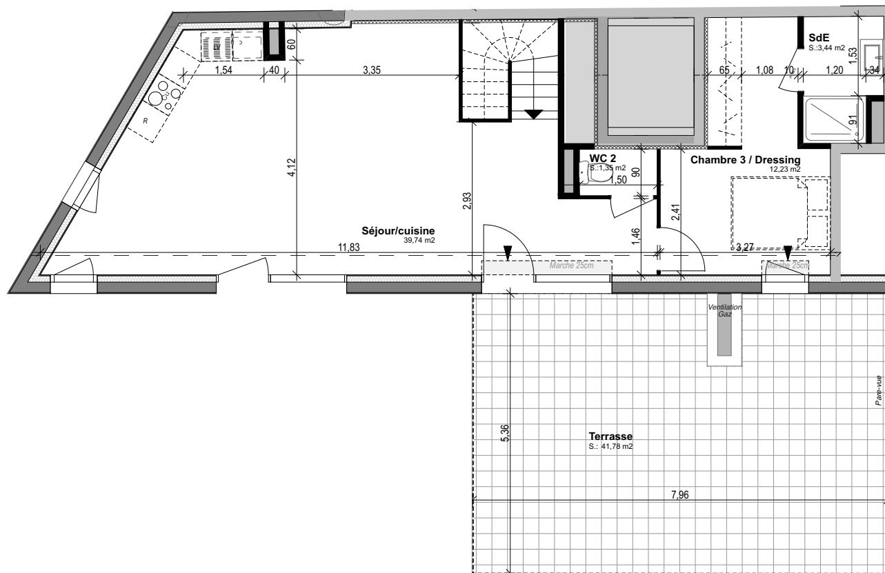
Plan du logement
